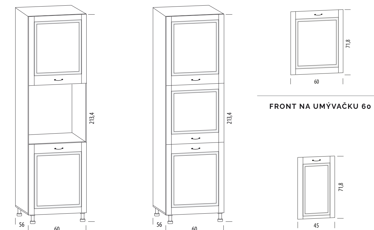
KORPUS 60H B CABINET A KORPUS 60H B CABINET B FRONT NA UMÝVAČKU 60
